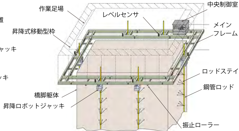
昇降式移動型枠・作業足場全体概念図
