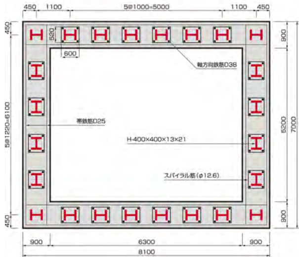
断面図（P2、P3）
