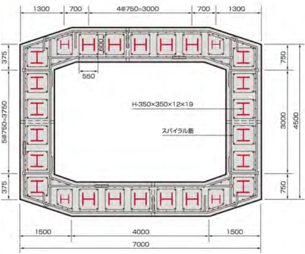
断面図（P1、P2）
