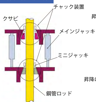
昇降口ボットジャッキ
