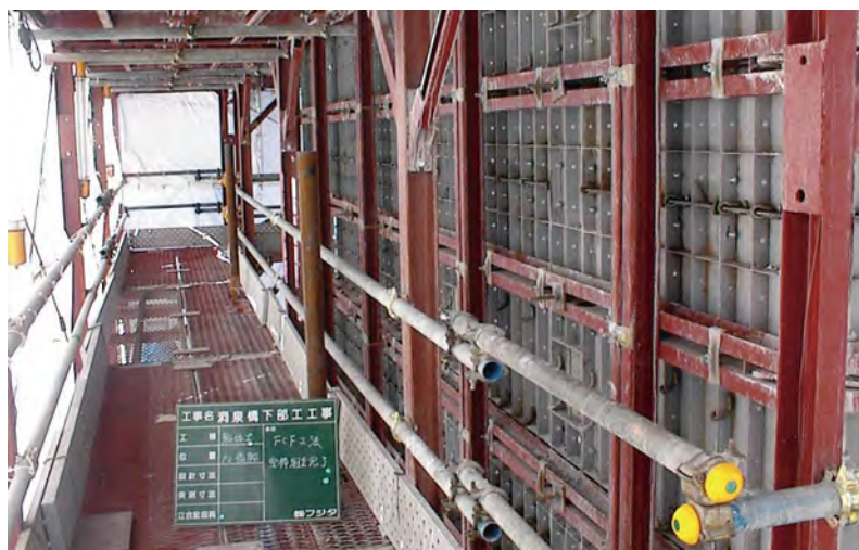
昇降式移動型枠 (外側)
