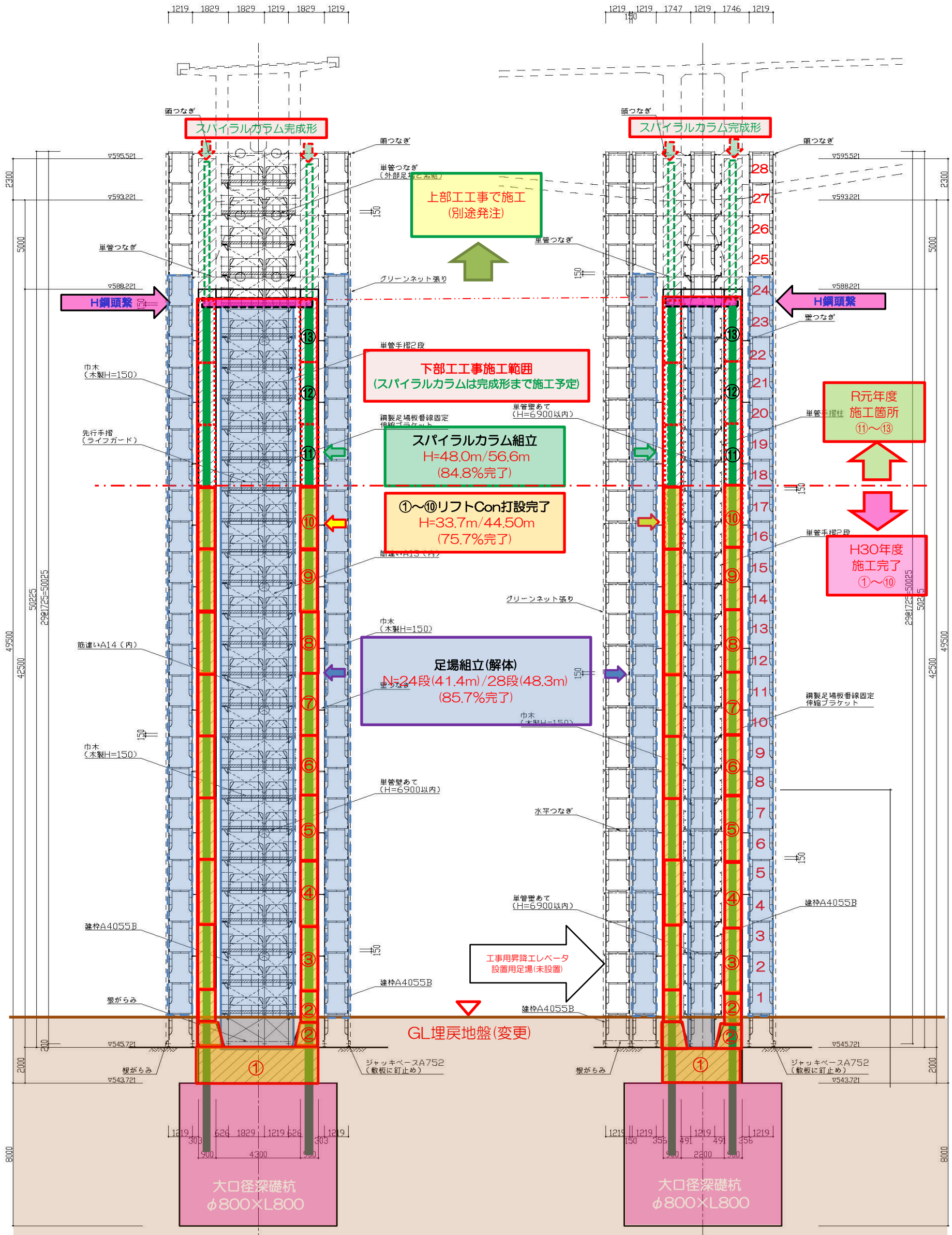
A-A断面図 1/100
