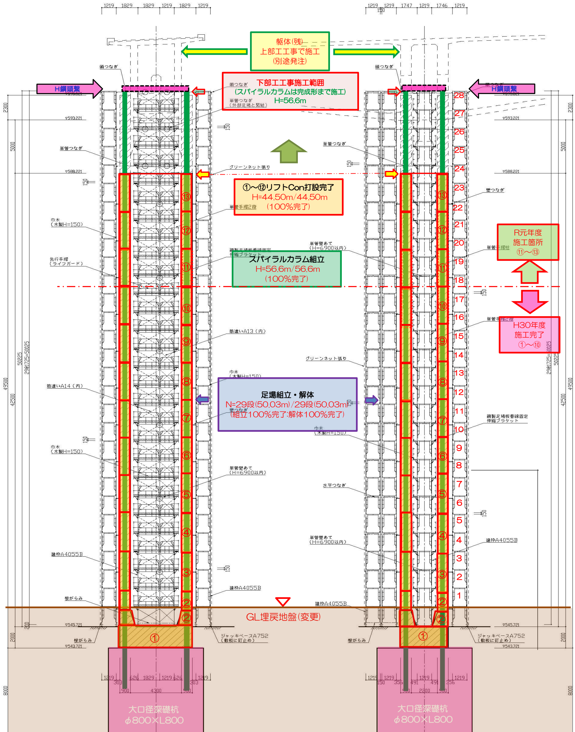
A-A断面図 1/100
